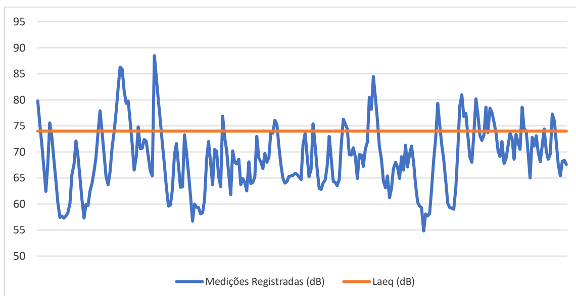
Figura 23- Comportamento do ruído no ponto amostral 02. Fonte: RIBAS Consultoria Ambiental, 2024.
