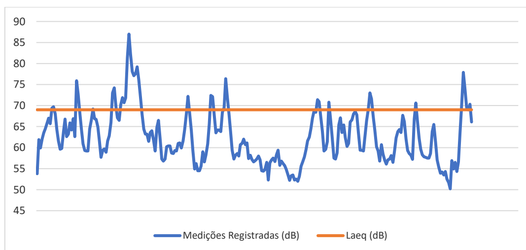
Figura 22- Comportamento do ruído no ponto amostral 01. Fonte: RIBAS Consultoria Ambiental, 2024.
